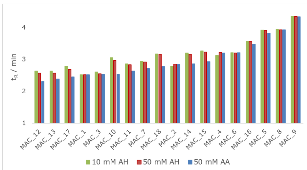
Slika 5.17 Usporedba vremena zadržavanja makrocikličkih spojeva dobivenih upotrebom amonijevog acetata koncentracije 50 mM (plavi stupci) te amonijevog hidrogenkarbonata koncentracije 50 mM (crveni stupci) odnosno 10 mM (zeleni stupci) kao puferske otopine korištene kao vodeni dio pokretne faze upotrebom Luna C18 kromatografske kolone (AA – amonijev acetat, AH – amonijev hidrogenkarbonat).
