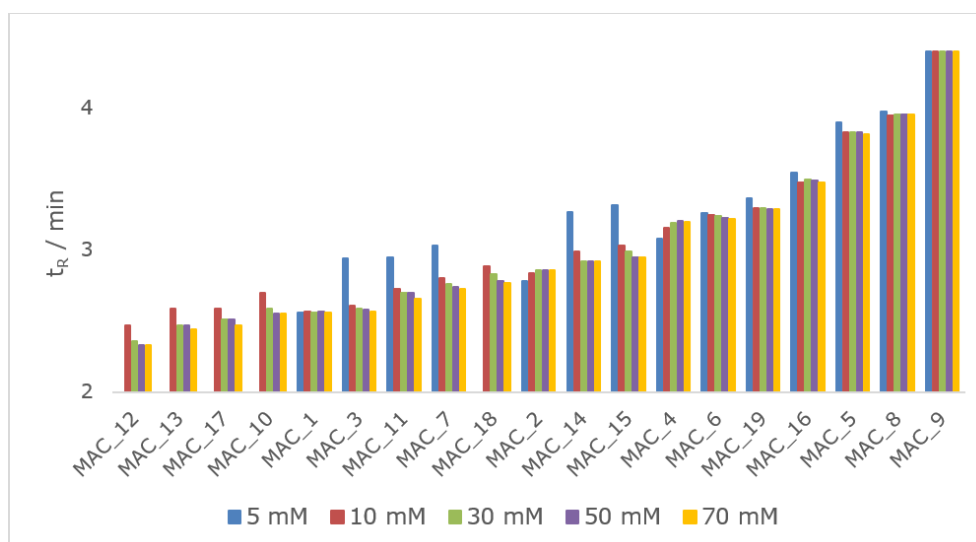
Slika 5.10 Usporedba vremena zadržavanja makrocikličkih spojeva dobivenih upotrebom amonijevog acetata koncentracije 5 mM (plavi stupci), 10 mM (crveni stupci), 30 mM (zeleni stupci), 50 mM (ljubičasti stupci) i 70 mM (žuti stupci) kao puferske otopine korištene kao vodeni dio pokretne faze na Luna C18 kromatografskoj koloni.
