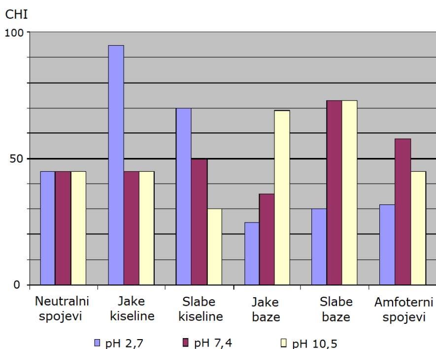
Slika 2.8 Kategorizacija spojeva ovisno o njihovom kiselobaznom karakteru pomoću CHI vrijednosti ovisno o pH vrijednosti puferne otopine korištene kao vodeni dio pokretne faze. Preuzeto i prilagođeno prema izvoru (105).
