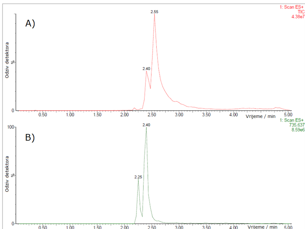
Slika 5.15 Kromatografski pikovi MAC_13 – azahomoeritromicin dobiveni upotrebom A) 5 mM i B) 70 mM amonijevog acetata kao puferske otopine korištene kao vodeni dio pokretne faze na XSelect kromatografskoj koloni.
