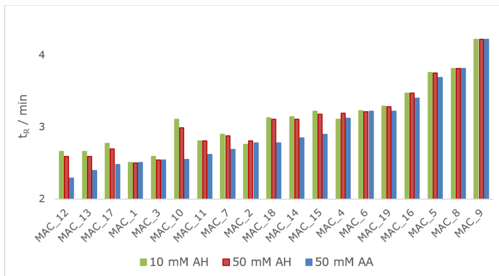
Slika 5.18 Usporedba vremena zadržavanja makrocikličkih spojeva dobivenih upotrebom amonijevog acetata koncentracije 50 mM (plavi stupci) te amonijevog hidrogenkarbonata koncentracije 50 mM (crveni stupci) i 10 mM (zeleni stupci) kao puferske otopine korištene kao vodeni dio pokretne faze na XSelect CSH kromatografskoj koloni (AA – amonijev acetat, AH – amonijev hidrogenkarbonat).
