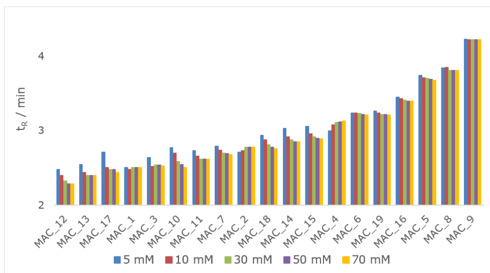
Slika 5.13 Usporedba vremena zadržavanja makrocikličkih spojeva dobivenih upotrebom amonijevog acetata koncentracije 5 mM (plavi stupci), 10 mM (crveni stupci), 30 mM (zeleni stupci), 50 mM (ljubičasti stupci) i 70 mM (žuti stupci) kao puferne otopine korištene kao vodeni dio pokretne faze na XSelect CSH kromatografskoj koloni.
