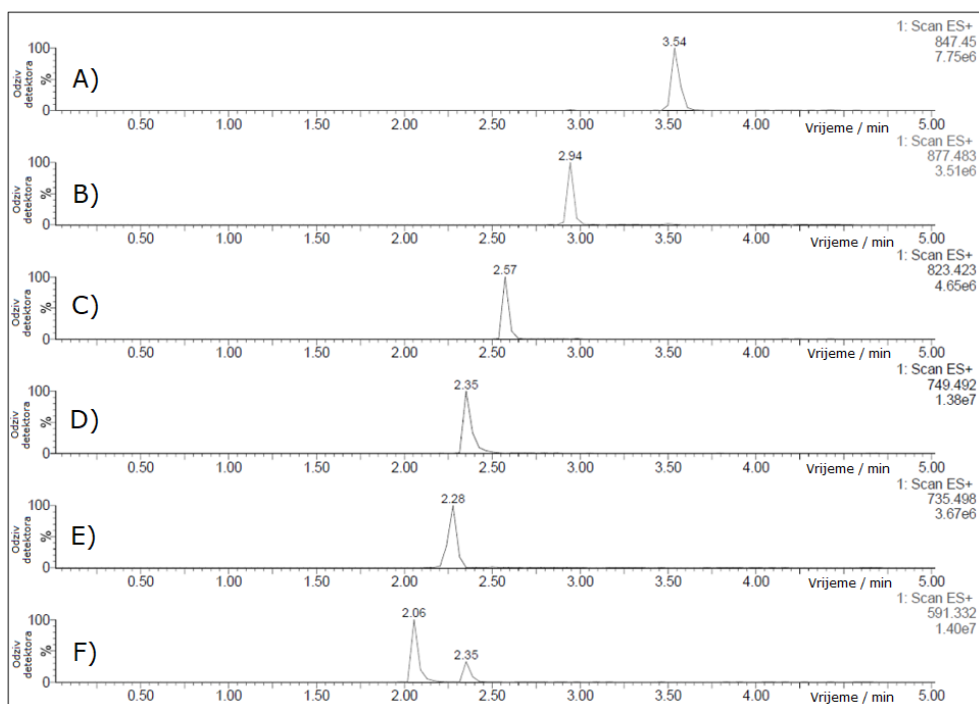
Slika 5.28 Kromatogrami dobiveni iz TIC kromatograma odabirom odgovarajuće m/z vrijednosti koja odgovara ionu odabranog standarda.
