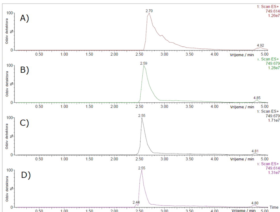
Slika 5.11 Kromatografski pikovi MAC_10 – azitromicina dobiveni upotrebom amonijevog acetata koncentracije A) 10 mM, B) 30 mM, C) 50 mM i D) 70 mM kao puferske otopine korištene kao vodeni dio pokretne faze na Luna C18 kromatografskoj koloni.
