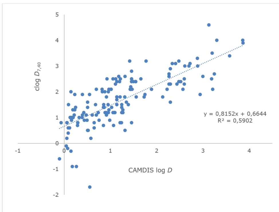
Slika 5.31 Korelacija između CAMDIS log D i \text{clog } D_{7,40} vrijednosti za proširenu skupinu makrocikličkih spojeva.
