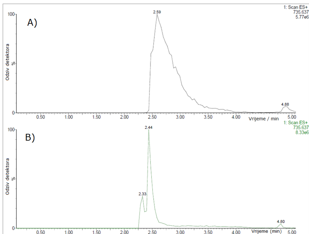
Slika 5.12 Kromatografski pikovi MAC_13 – azahomoeritromicina dobiveni upotrebom amonijevog acetata koncentracije A) 10 mM i B) 70 mM kao puferske otopine korištene kao vodeni dio pokretne faze na Luna C18 kromatografskoj koloni.
