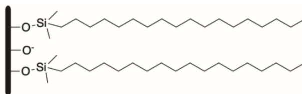
Slika 2.5 Oktadecil (C18) nepokretna faza vezana na silikagel. Preuzeto i prilagođeno prema izvoru (16).
