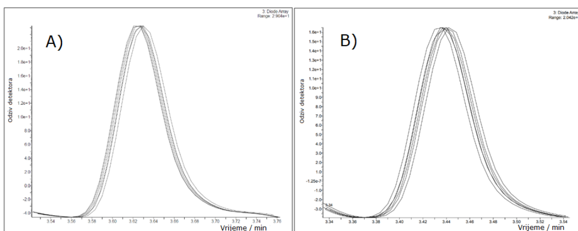
Slika 5.16 Vremena zadržavanja spojeva A) MAC_16 – josamicina i B) MAC_19 – midekamicina upotrebom amonijevog hidrogenkarbonata koncentracije 50 mM kao puferske otopine korištene kao vodeni dio pokretne faze u rasponu od 35 sati.
