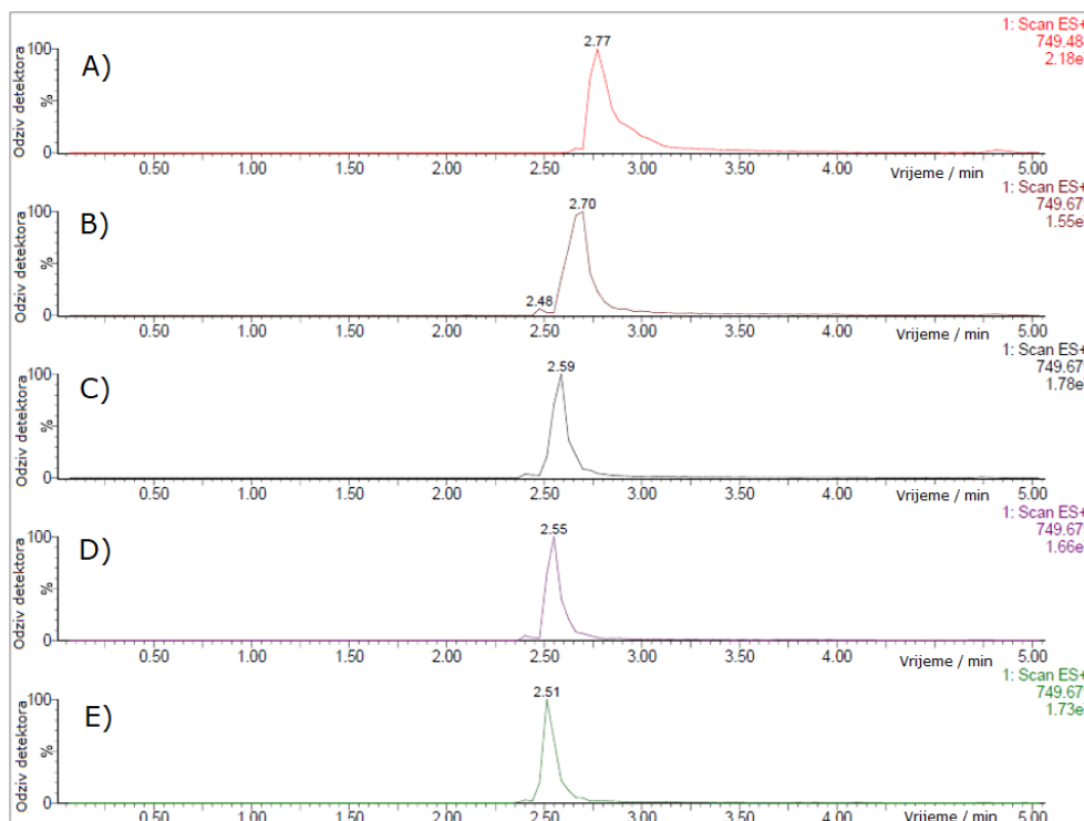
Slika 5.14 Kromatografski pikovi MAC_10 – azitromicina dobiveni upotrebom amonijevog acetata koncentracije A) 5 mM, B) 10 mM, C) 30 mM, D) 50 mM i E) 70 mM amonijevog acetata kao puferske otopine korištene kao vodeni dio pokretne faze na XSelect CSH kromatografskoj koloni.
